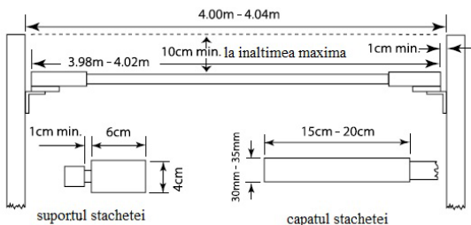
Figura TR27 – Tachetii și stacheta pentru săritura în înălțime
