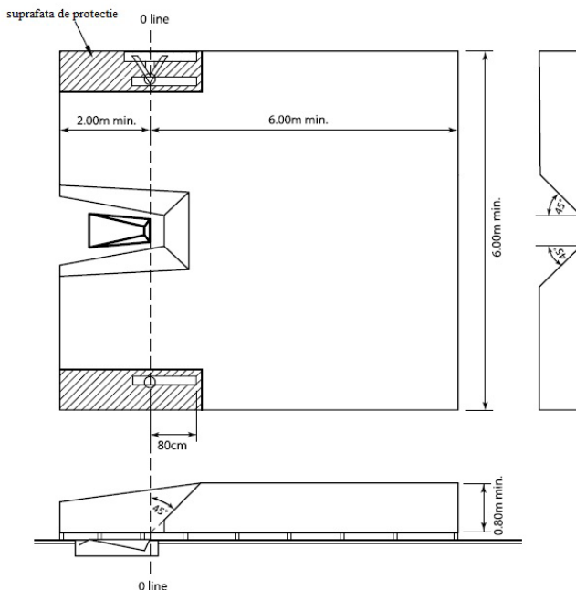
Figura (c) TR28 - Zona de aterizare a săriturii cu prăjină (vedere de sus și laterale)
