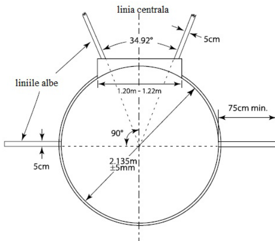
Figura (a) TR32 - Dispunerea cercului de aruncare a greutății
