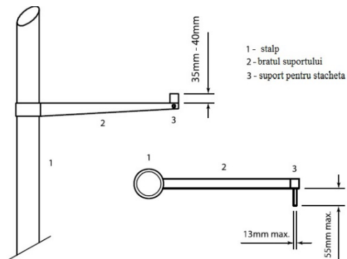
Figura (b) TR28 – Suportul șachteide la săritura cu prăjina (vedere din zona de aterizare și vedere de sus)
